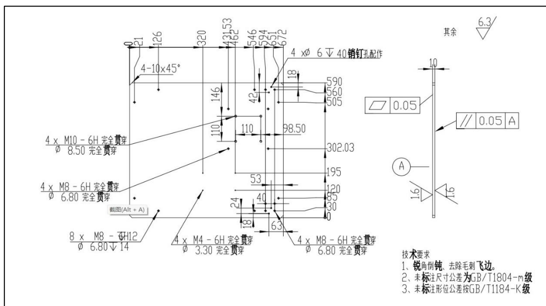
图 13：协作机器人固定钢板加工图纸 (仅供参考尺寸，不做加工要求)
