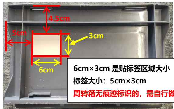
图 3：周转箱侧壁贴标签位置
