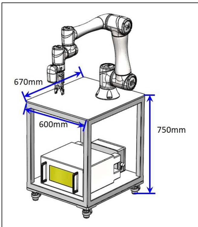
图 11：协作机器人底座
